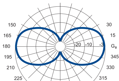
Диаграмма направленности в вертикальной плоскости
