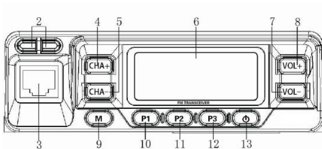
Передняя панель
