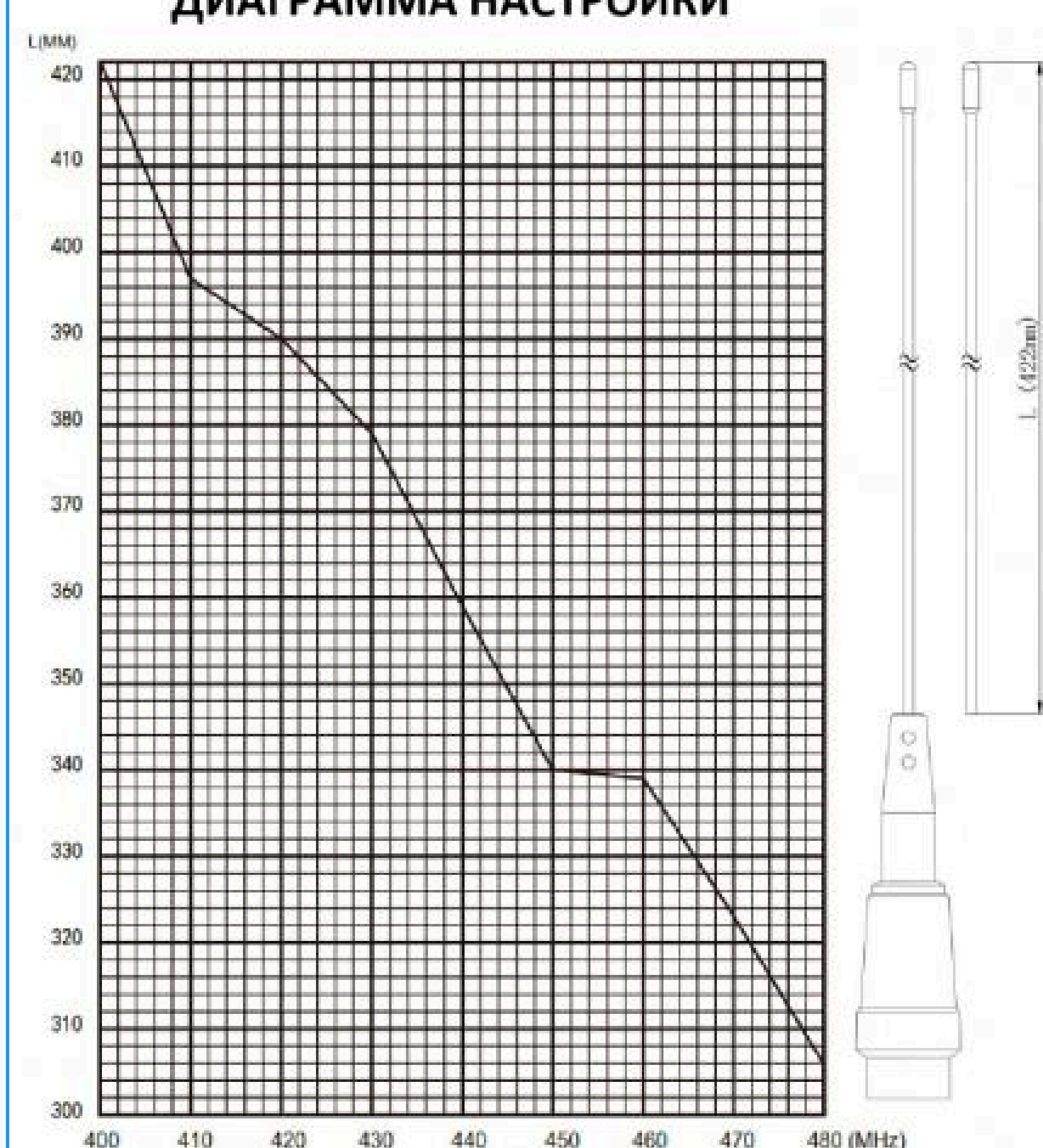
ДИАГРАММА НАСТРОЙКИ
