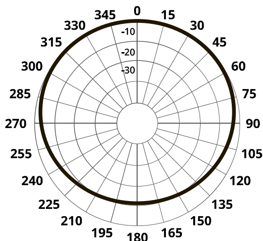
RA-DP1U в H-плоскости
