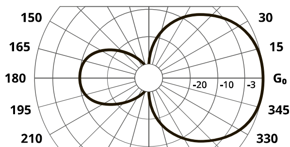
RA-DP1U в E-плоскости
