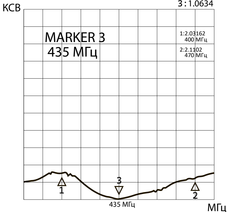
ГРАФИК КСВ
