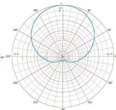
H-Plane | 425 MHz
