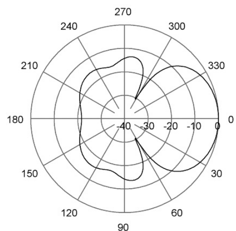
H-Plane | 165 MHz
