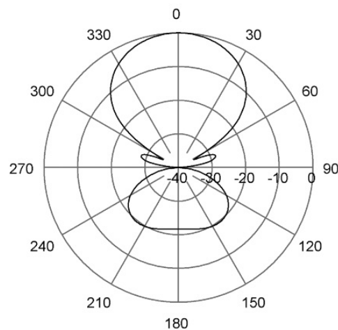
E-Plane | 165 MHz
