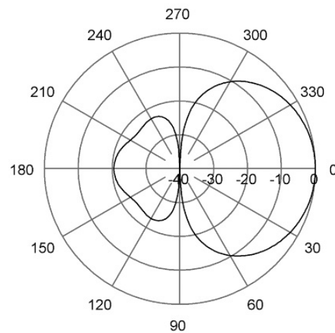
E-Plane | 165 MHz
