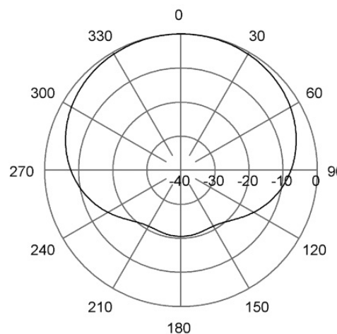
H-Plane | 165 MHz
